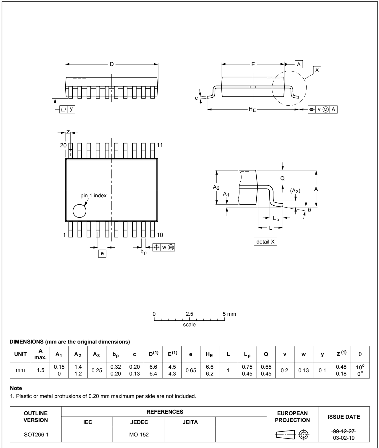
Fig. 1. Package outline SSOP20 (SOT266-1)
